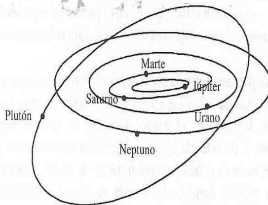
Todos los planetas, satélites, asteroides, etc., de un sistema solar, describen órbitas elípticas.
